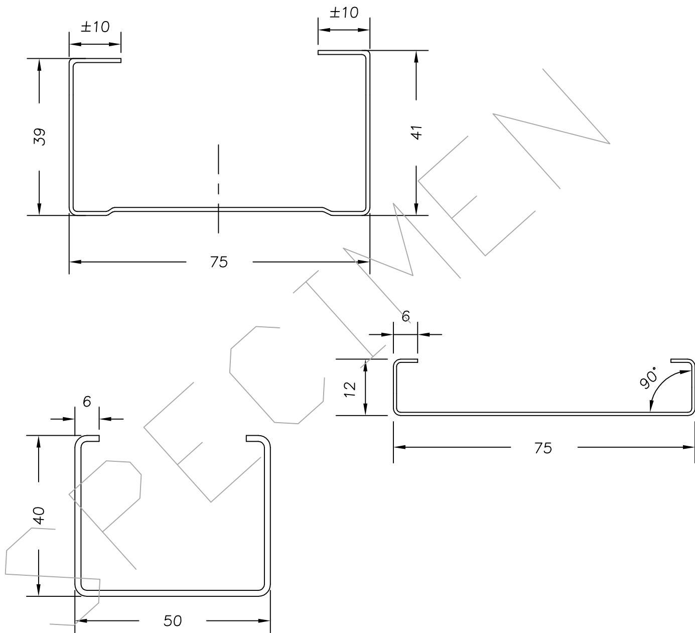
C-Profiel
